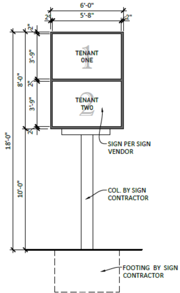
PYLON SIGN 9 SCALE: 1/4" = 1'-0"
