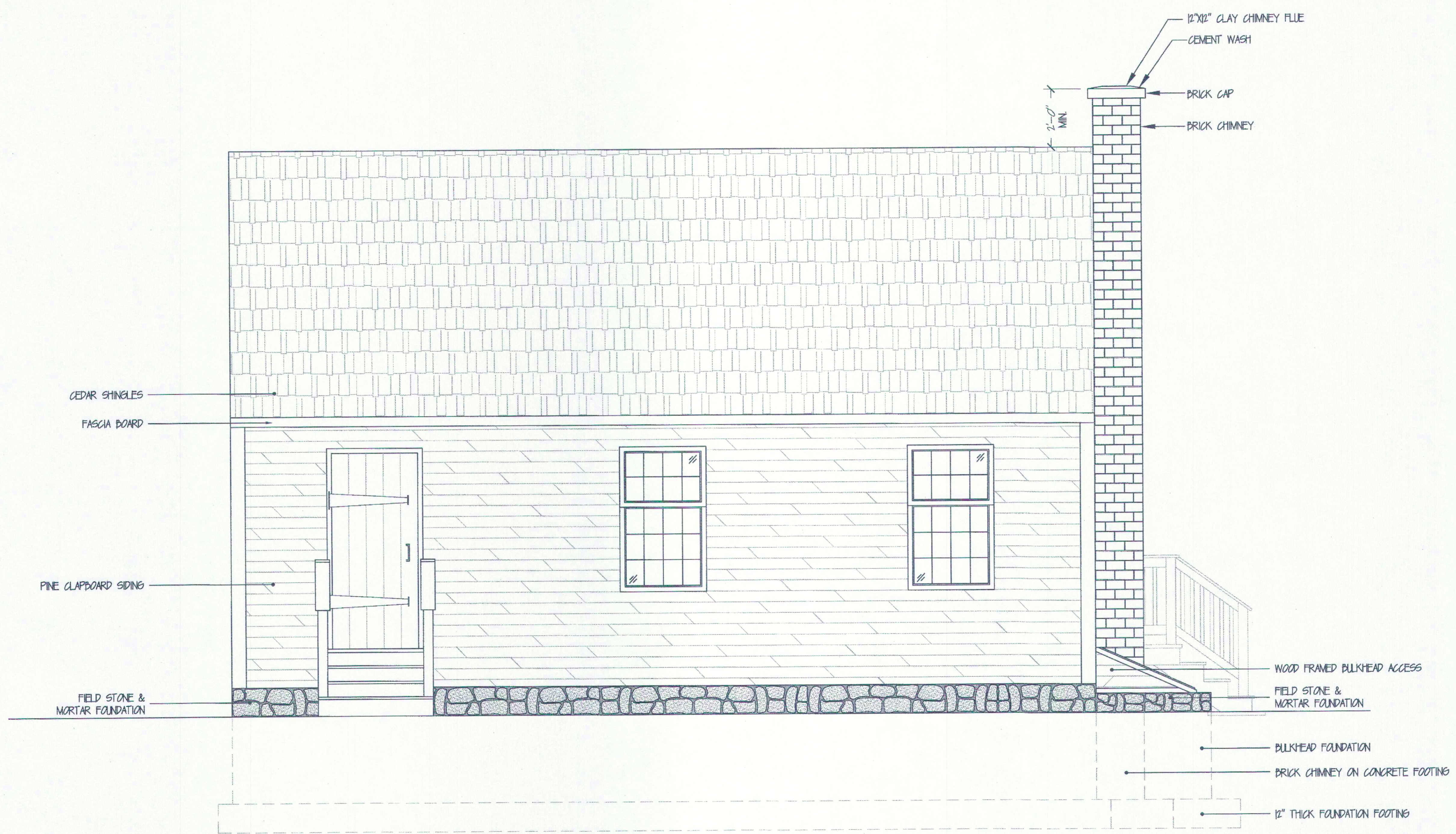
1 NORTH ELEVATION A5 SCALE: 1/2"=1'-0"
